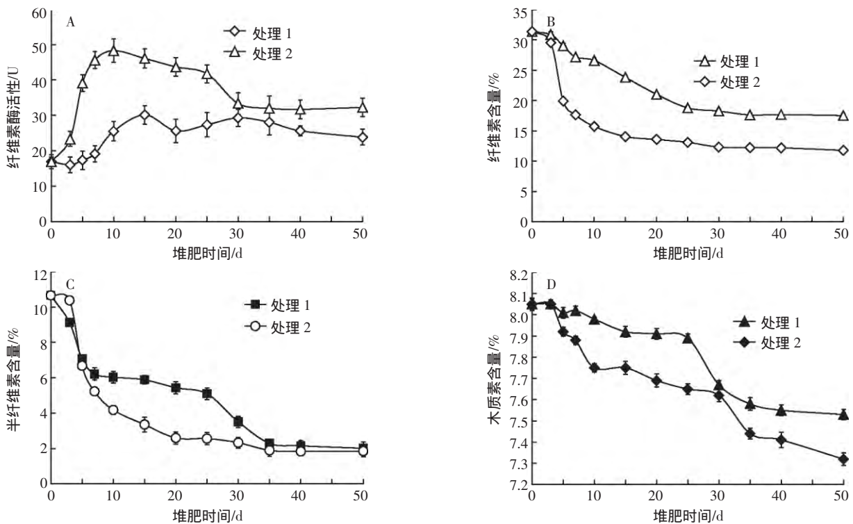
图2 木薯渣堆肥过程中纤维素酶活性以及纤维素、半纤维素和木质素的变化
