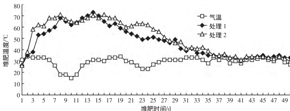
图1 木薯渣堆肥过程中温度变化
