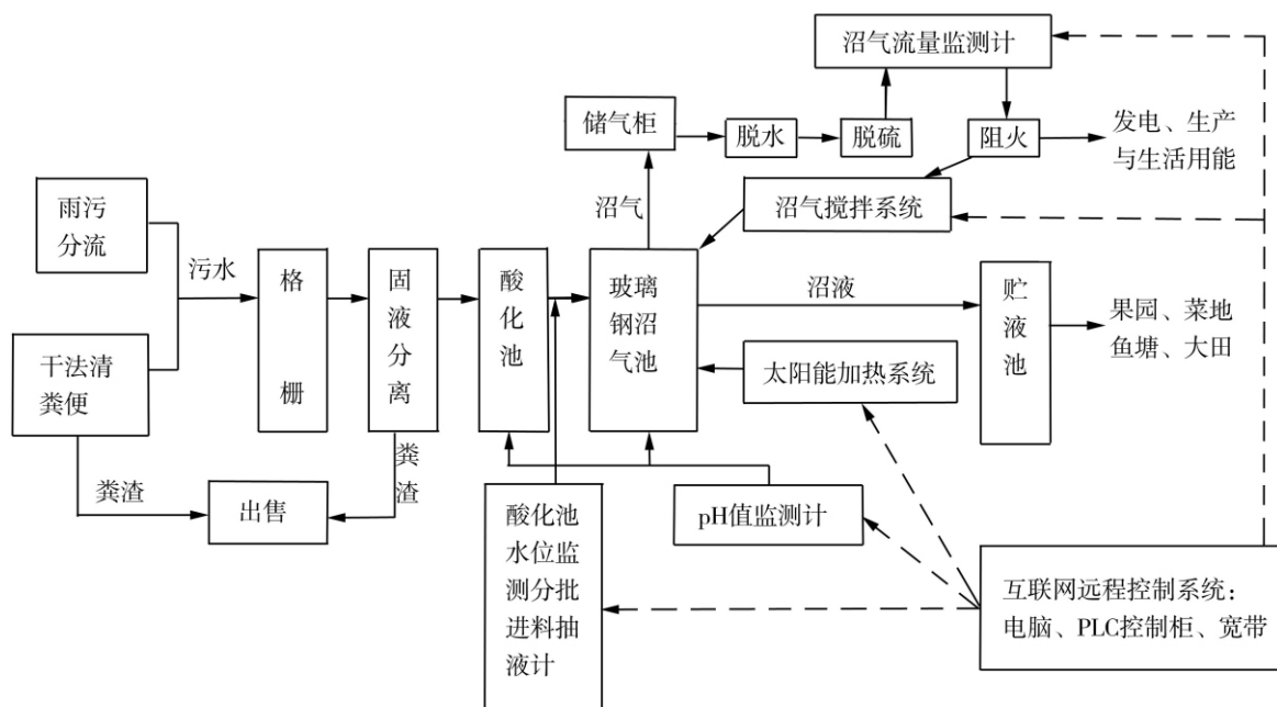
图1 智能化沼气工程的工艺运行流程
