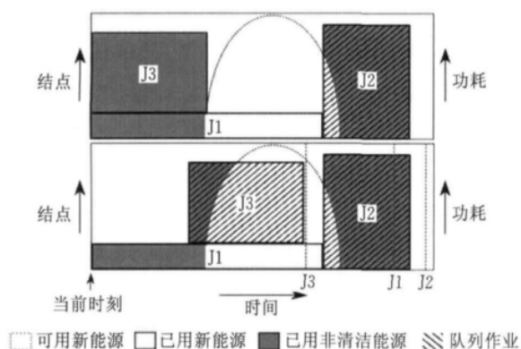
图3 在调度3个作业(J1, J2, J3)时, 回填(Backfill)算法(上图)与 GreenSlot(下图)算法的对比.
