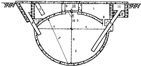
1—水压酸化池；2—发酵主池；3—储气箱；4—进料管；5—出料管；6—活动盖；
