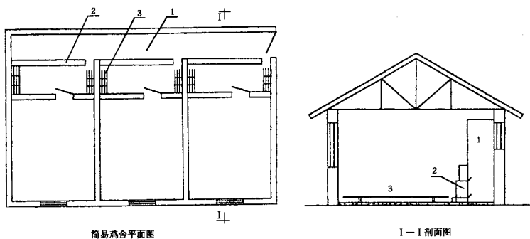
1—走道;2—产蛋箱;3—栖架 图 D1 简易鸡舍结构示意图
