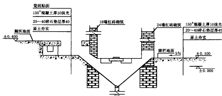
图 A4 强回流三结合沼气池 II—II 剖面图
