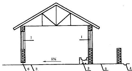
1—通风窗;2—食槽;3—猪床;4—沟道;5—运动场;6—溢流口
