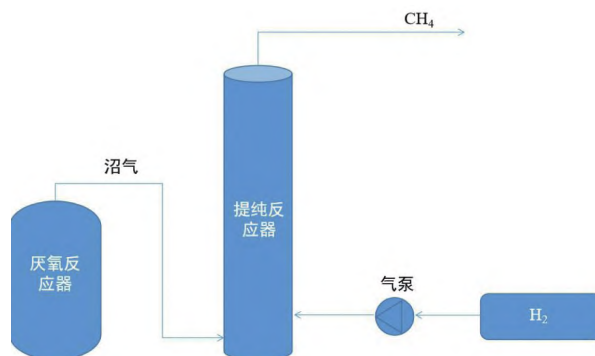
图7 CO 2 异位利用技术工艺流程示意图
