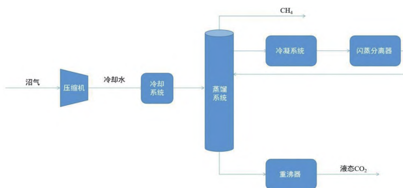
图4 低温分离技术工艺流程示意图
