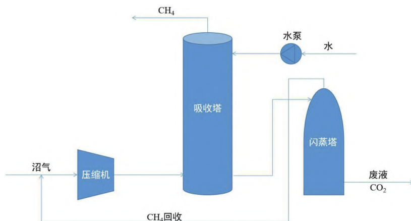
图2 水洗技术工艺流程示意图
