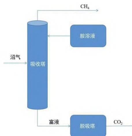
图5 化学吸收技术工艺流程示意图
