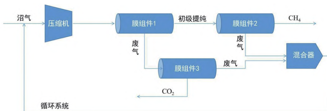
图1 膜分离技术工艺流程示意图
