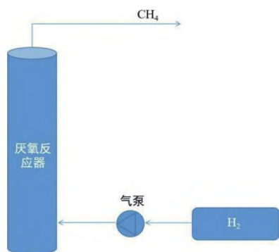
图6 CO 2 原位利用技术工艺流程示意图
