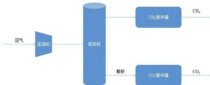
图3 变压吸附技术工艺流程示意图
